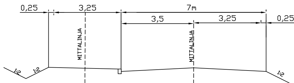
Reunakivellinen poikkileikkaus
