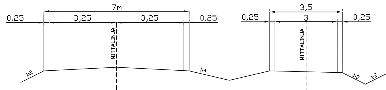
Väliskaistallinen poikkileikkaus
